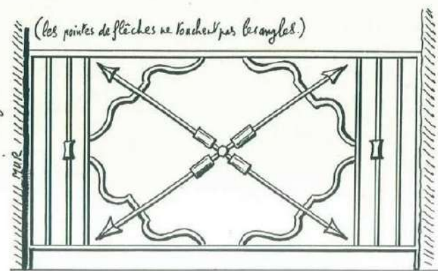
balustrade sous fenêtre.
